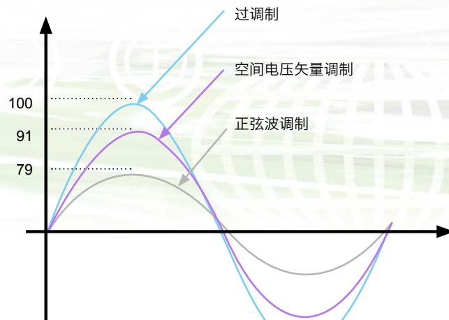
过调制技术
